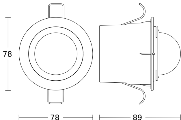
Dibujo acotado
