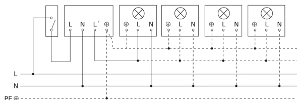
Diagrama electrónico lámpara con conductor neutro
