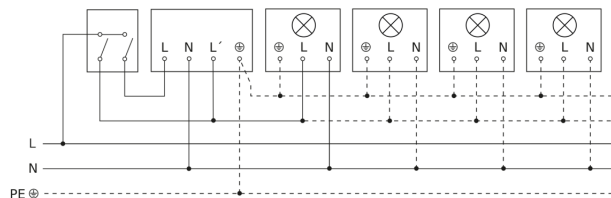
Diagrama electrónico conexión mediante interruptor en serie para funcionamiento manual y automático
