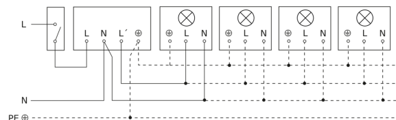
Diagrama electrónico lámpara sin conductor neutro
